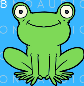
SAPO
