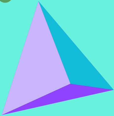
PIRÁMIDE TRIANGULAR
