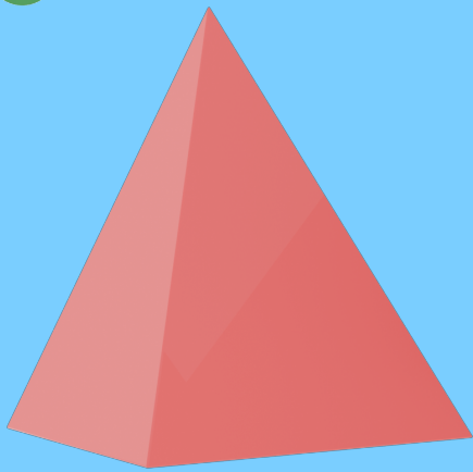
PIRÁMIDE CUADRANGULAR
