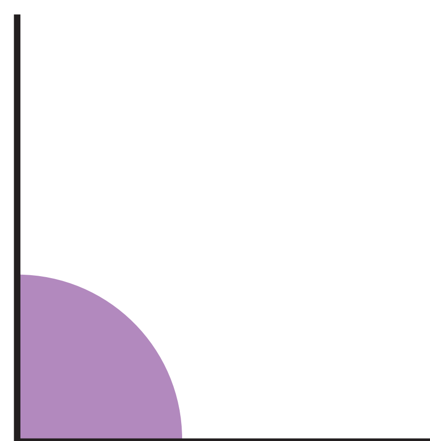
ÁNGULO RECTO
