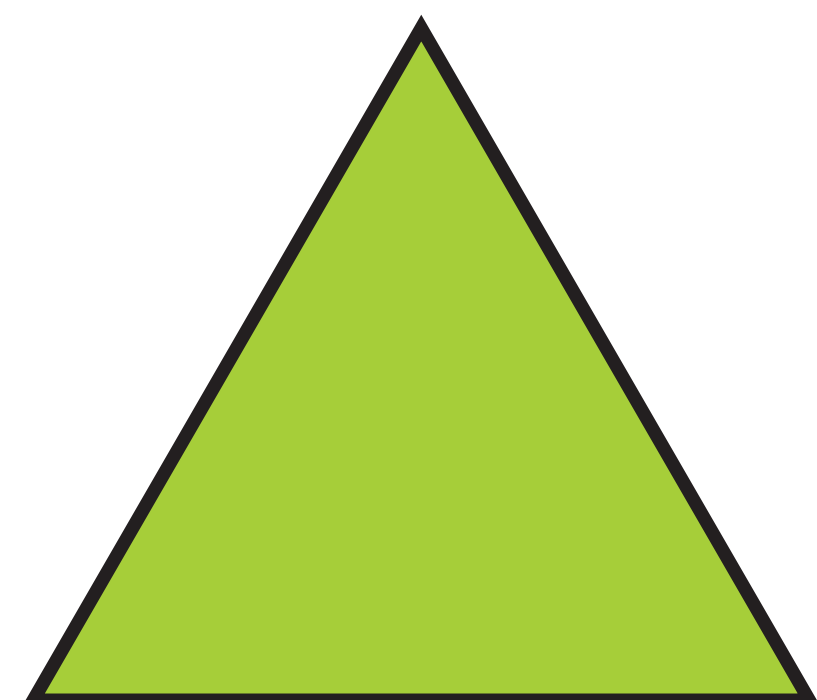
TRIÁNGULO
