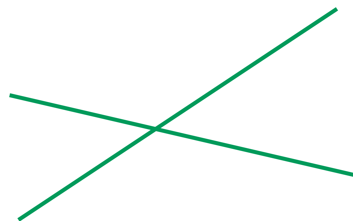
RECTAS SECANTES
