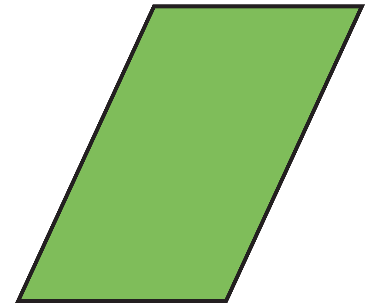
ROMBOIDE
