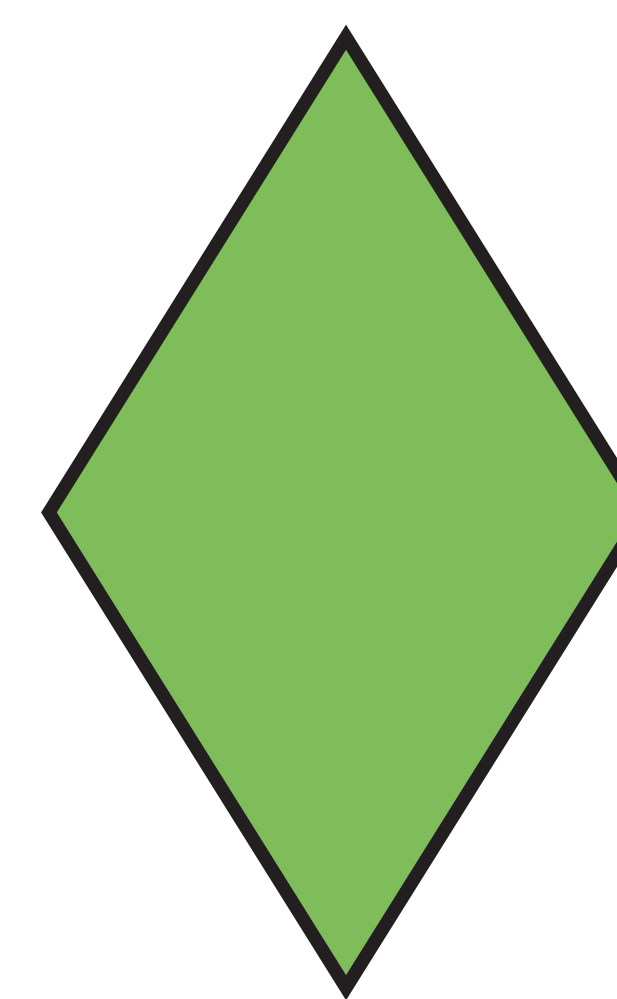
ROMBO
