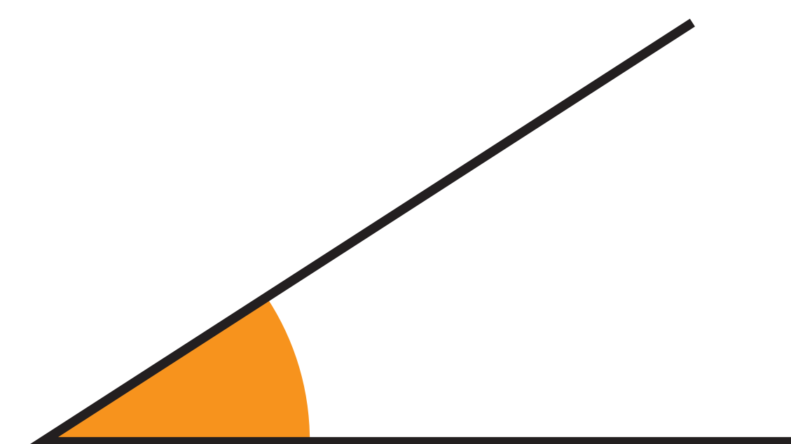
ÁNGULO AGUDO
