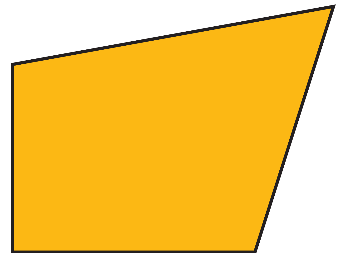
Trapezoide
