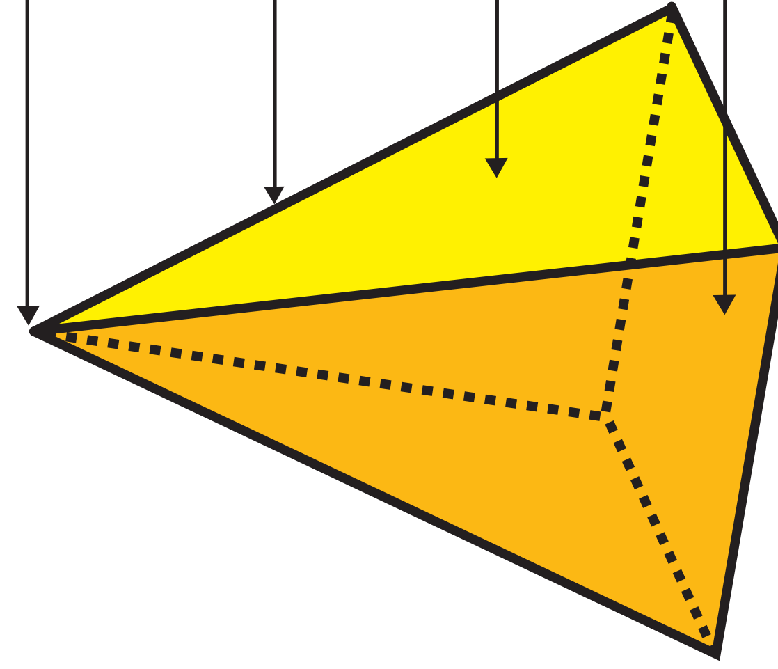
PIRÁMIDE CUADRANGULAR
