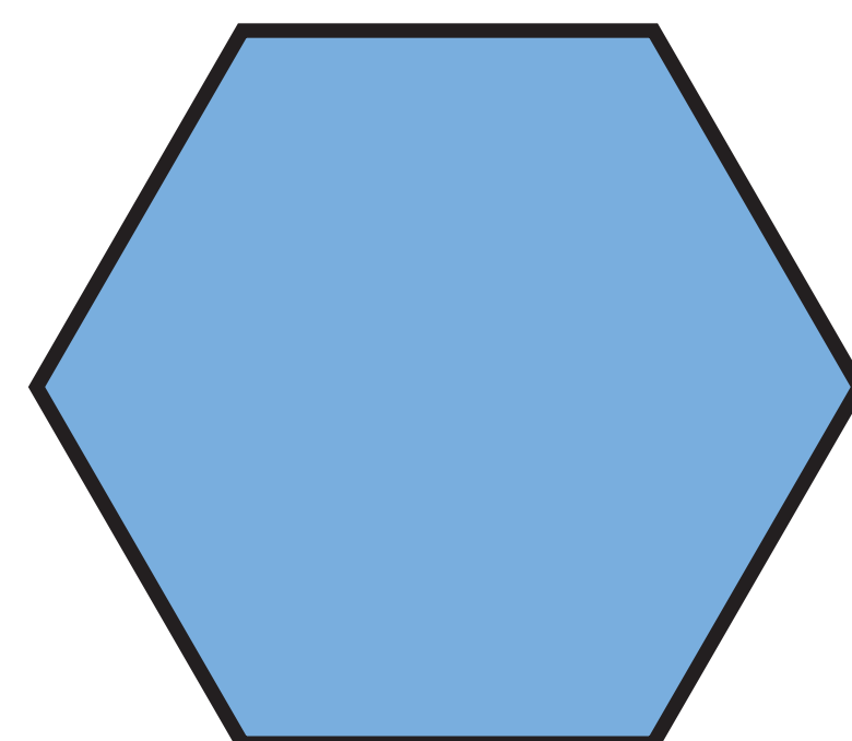
HEXÁGONO
