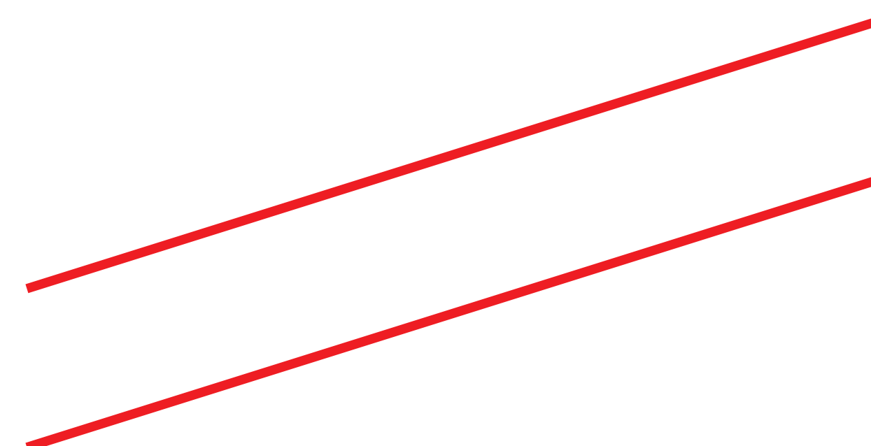
RECTAS PARALELAS
