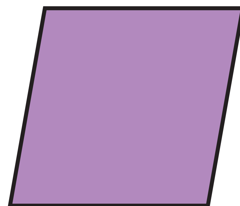
CUADRILÁTERO
