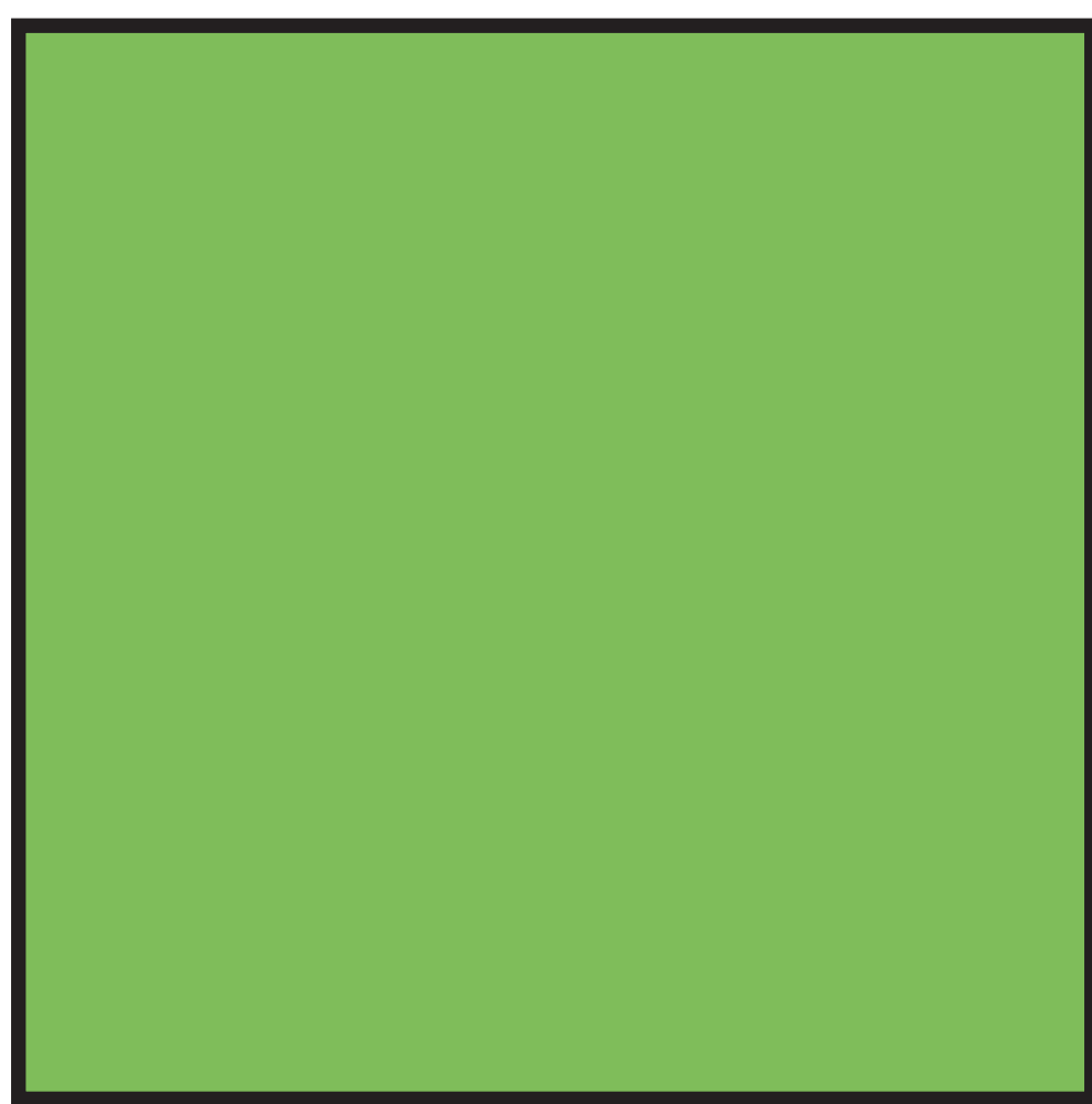
CUADRADO
