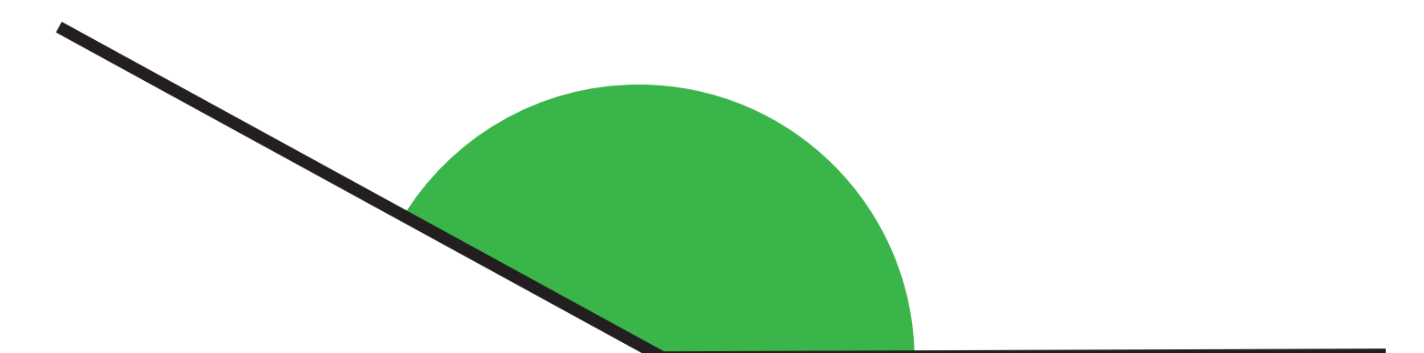
ÁNGULO OBTUSO
