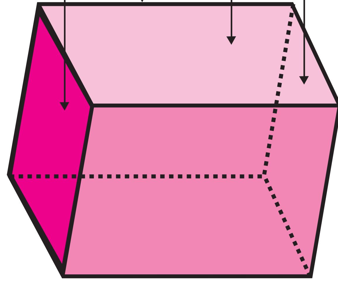
PRISMA CUADRANGULAR
