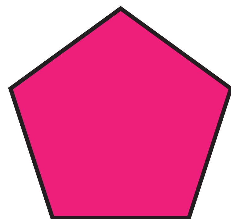
PENTÁGONO
