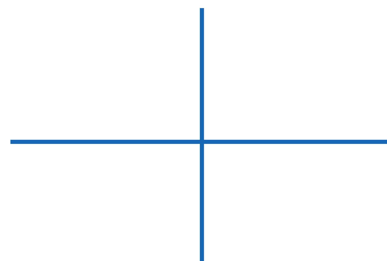
RECTAS PERPENDICULARES
